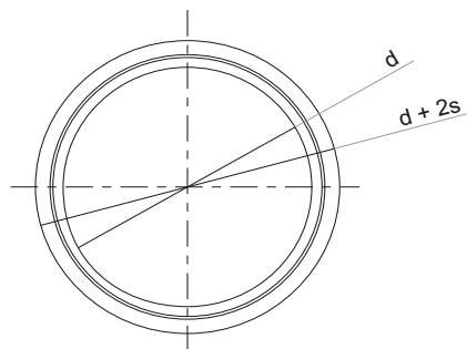
PRSTEN (nastavak) MONTAŽNOG REVIZIJSKOG OKNA KBS 8 s ugrađenom penjalicom
